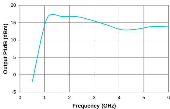
Output P1dB
