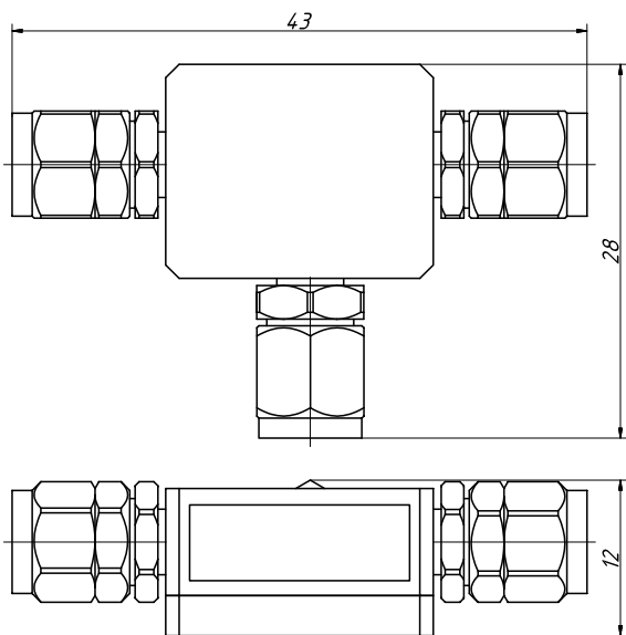
Смесители: 3,2 – 19,2/2; 3,2 – 19,2/4; 3 – 20/2; 5 – 26/2; 13 – 50/2.
