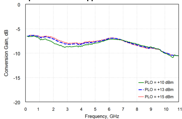
IF sweep to RF 4 GHz / Upper LO
