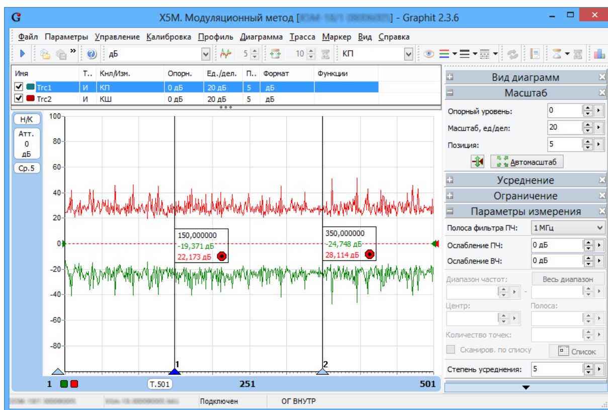
Рисунок 4.1 Внешний вид Graphit X5M со скрытым отображением частот
